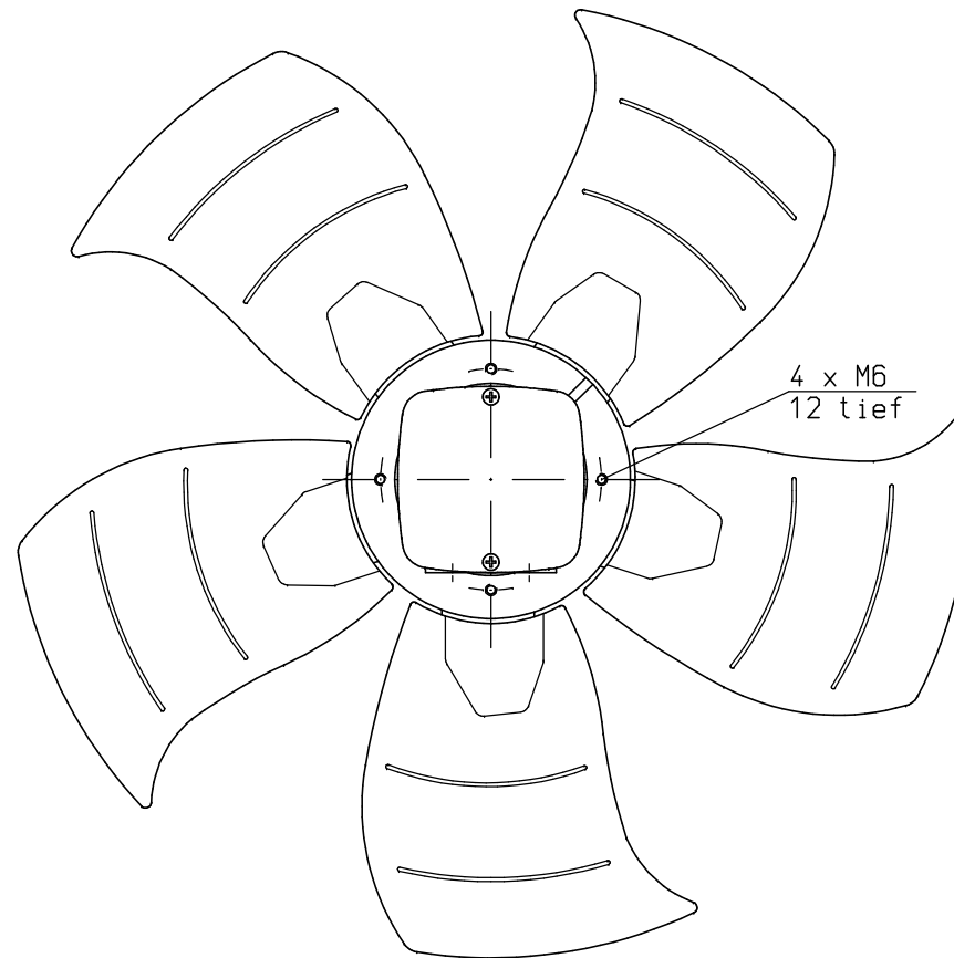
Ansicht ohne Tragegitter/view without guard
